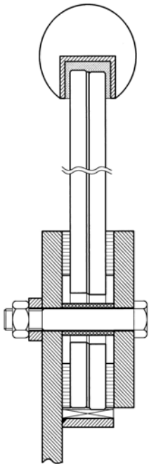
Schematische Darstellung, nicht maßstäblich
